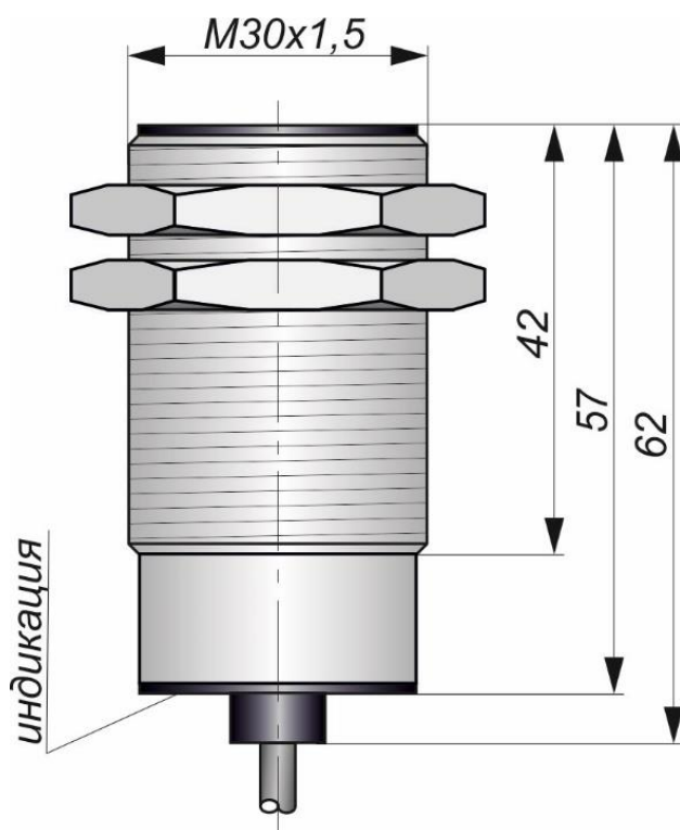
Габаритный чертеж
